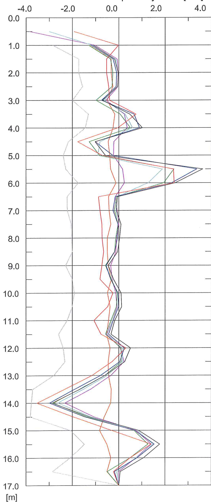
Przemieszczenia w płaszczyźnie E [mm]
