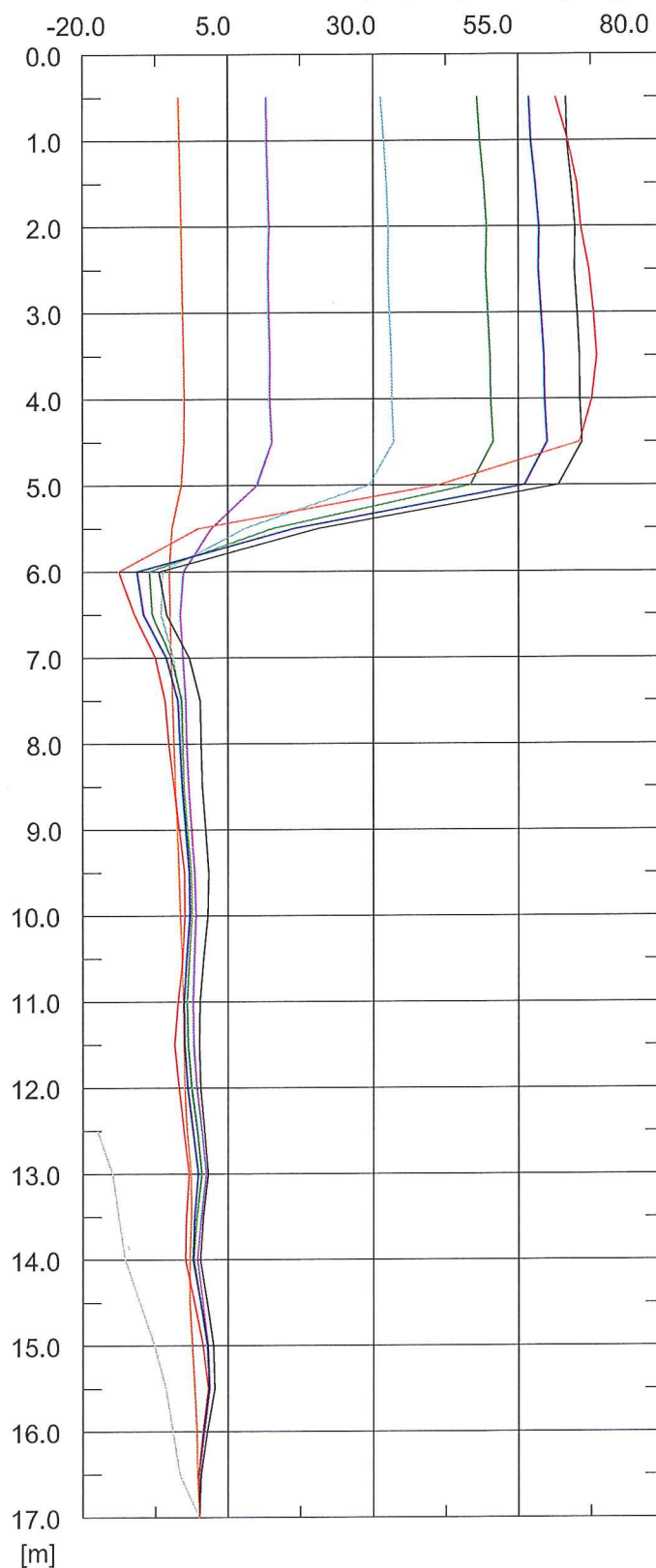
Przesunięcia w płaszczyźnie N [mm]
