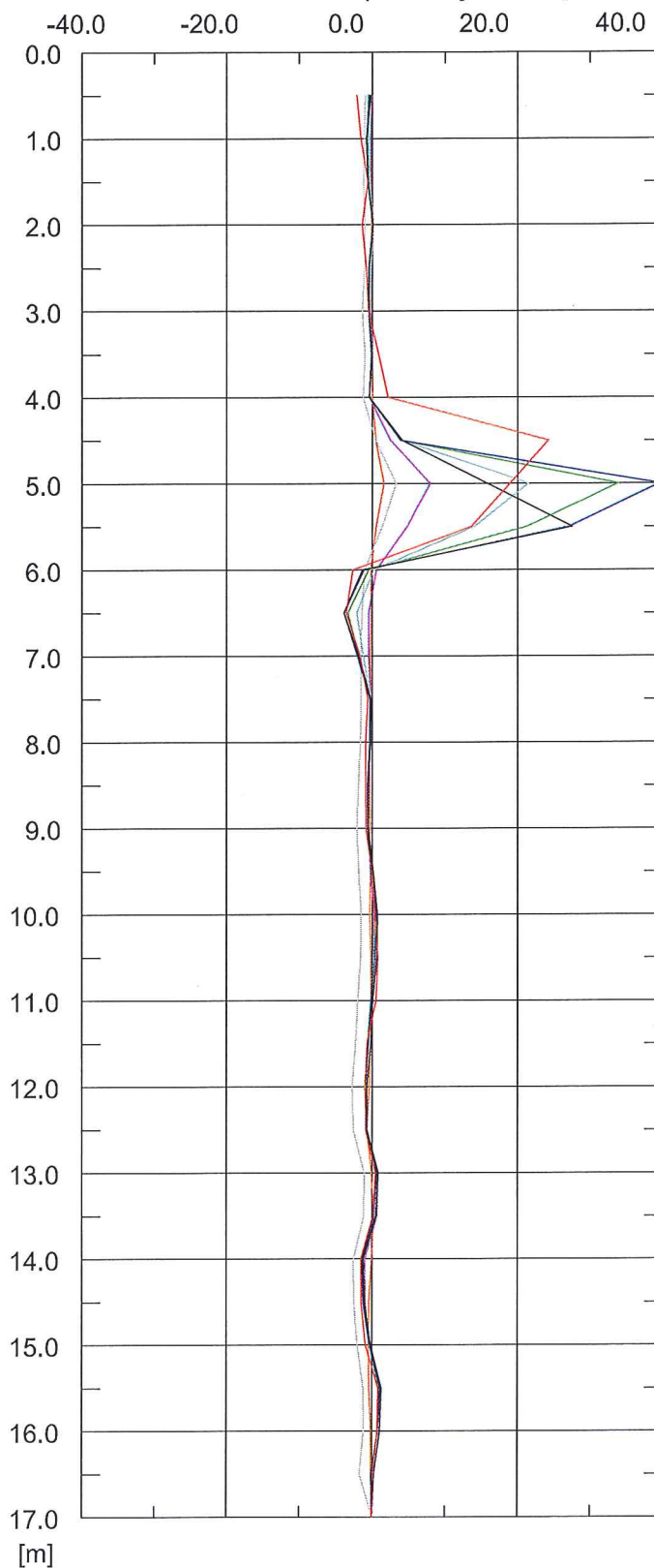
Przemieszczenia w płaszczyźnie N [mm]
