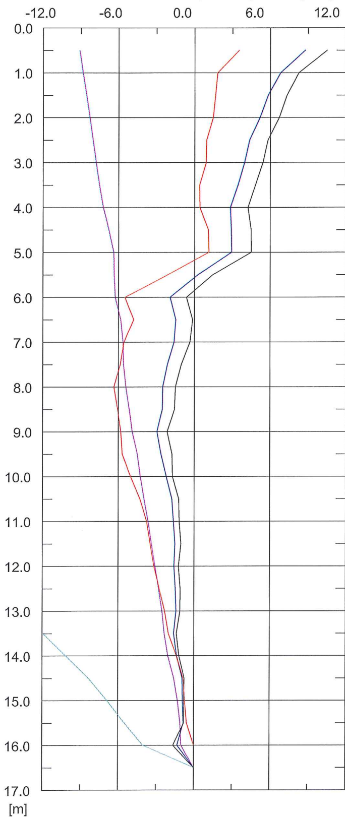
Przesunięcia w płaszczyźnie E [mm]
