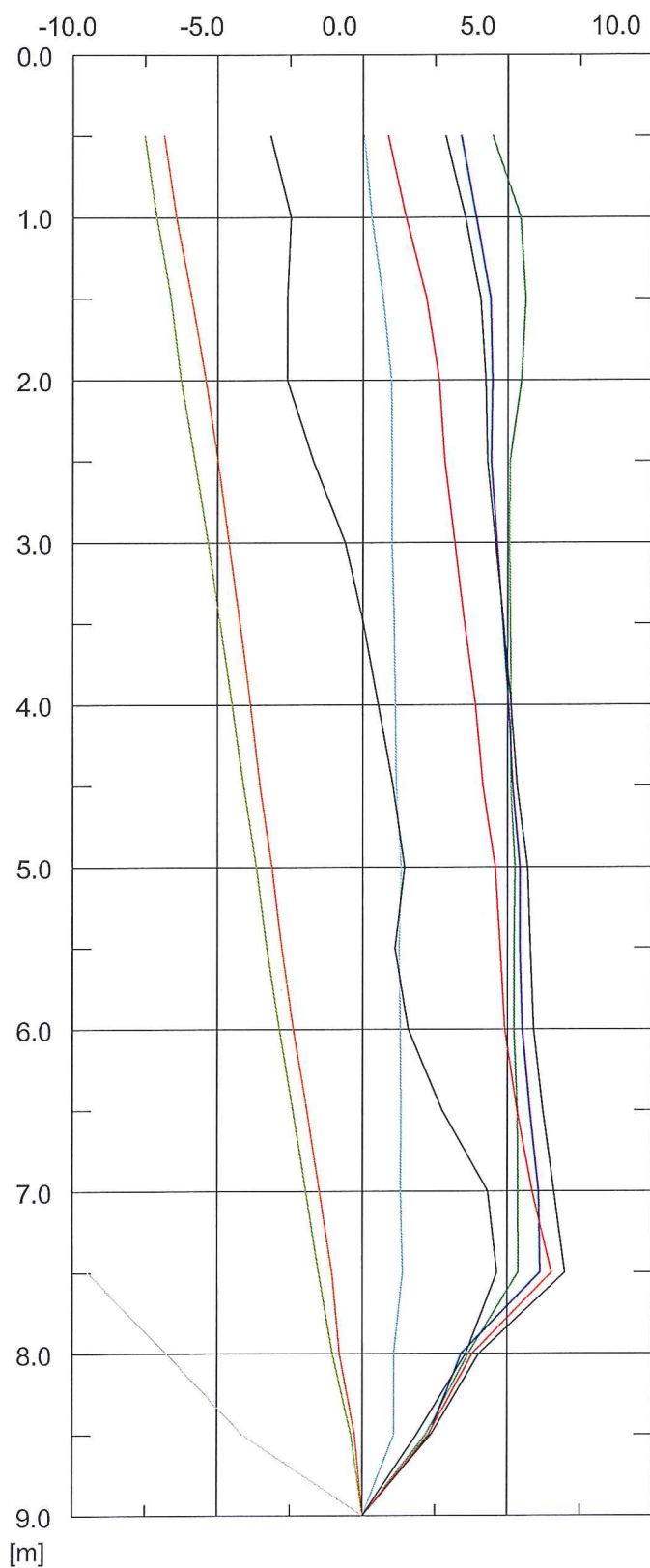
Przeszacowania w płaszczyźnie E [mm]
