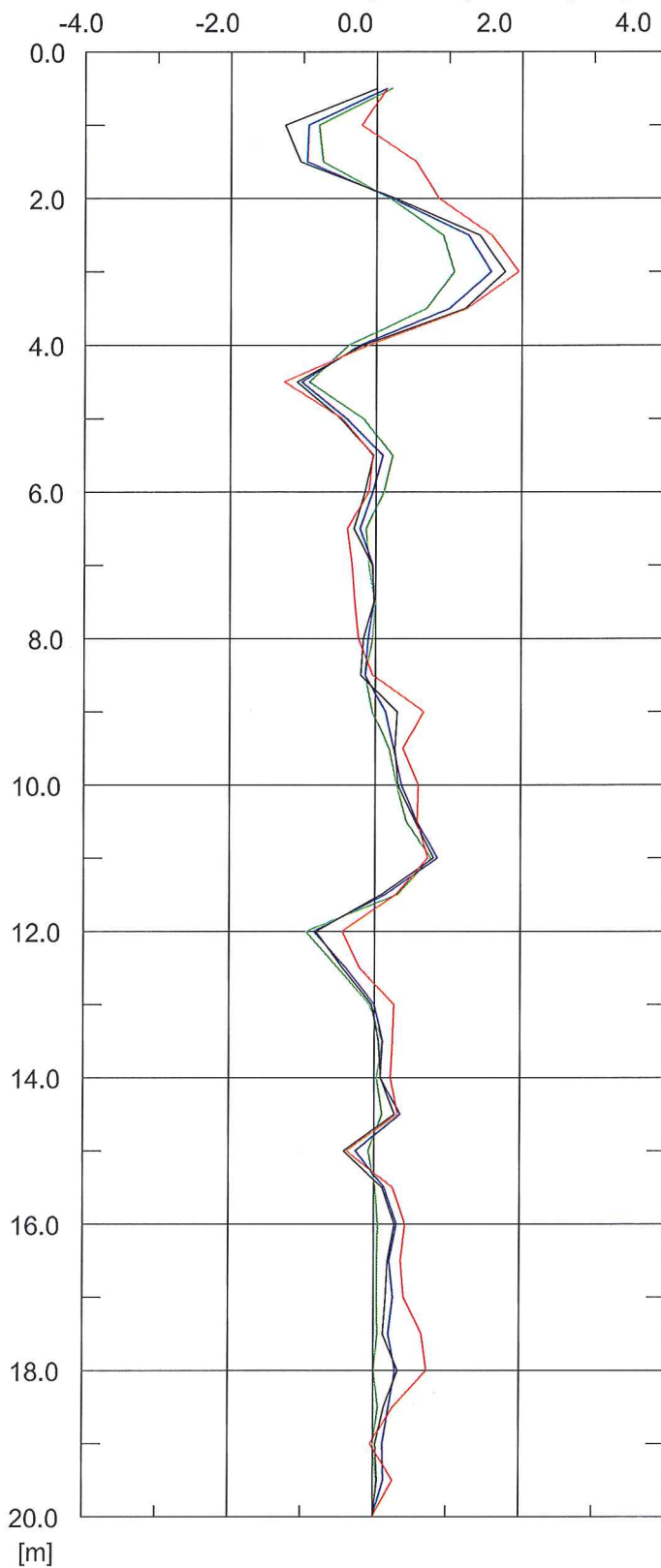
Przemieszczenia w płaszczyźnie N [mm]
