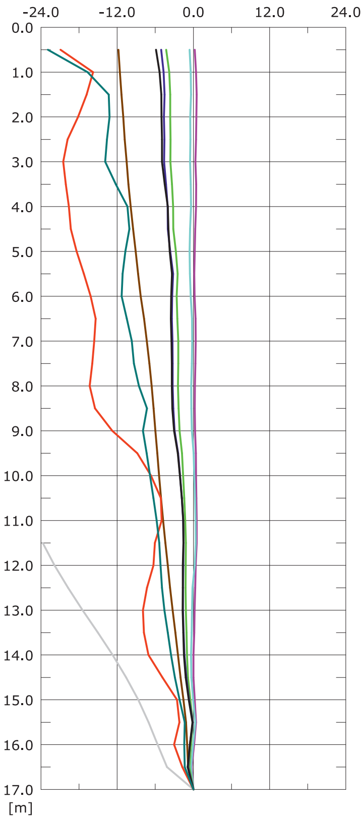
Przemieszczenia w płaszczyźnie E [mm]
