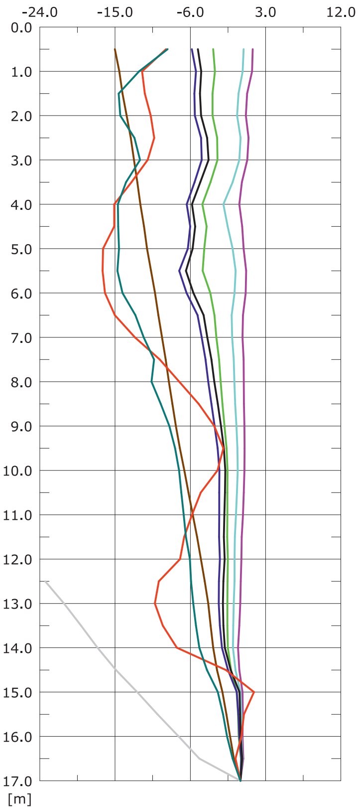
Przemieszczenia w płaszczyźnie N [mm]
