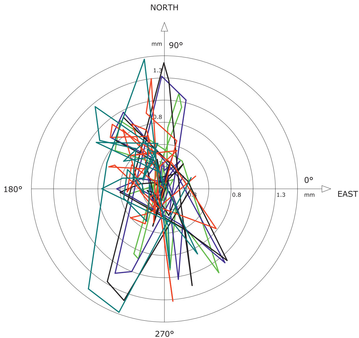
Wykres biegunowy przemieszczeń
