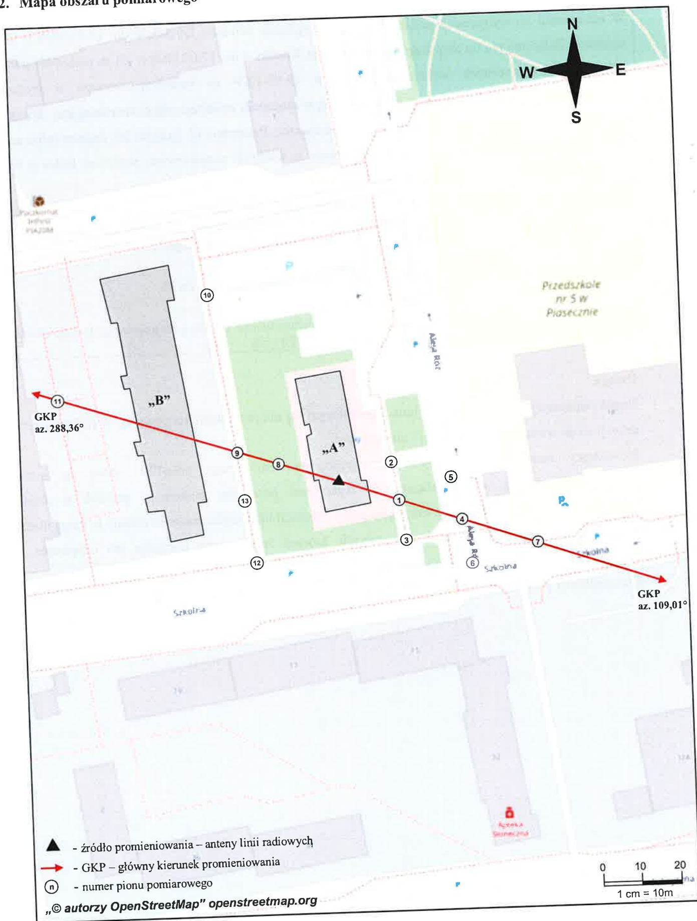
Rys. 1. Usytuowanie punktów i pionów pomiarowych w otoczeniu instalacji radiokomunikacyjnej Stacja Netia PIASB021-PIASM00004 Piaseczno, ul. Szkolna 20
