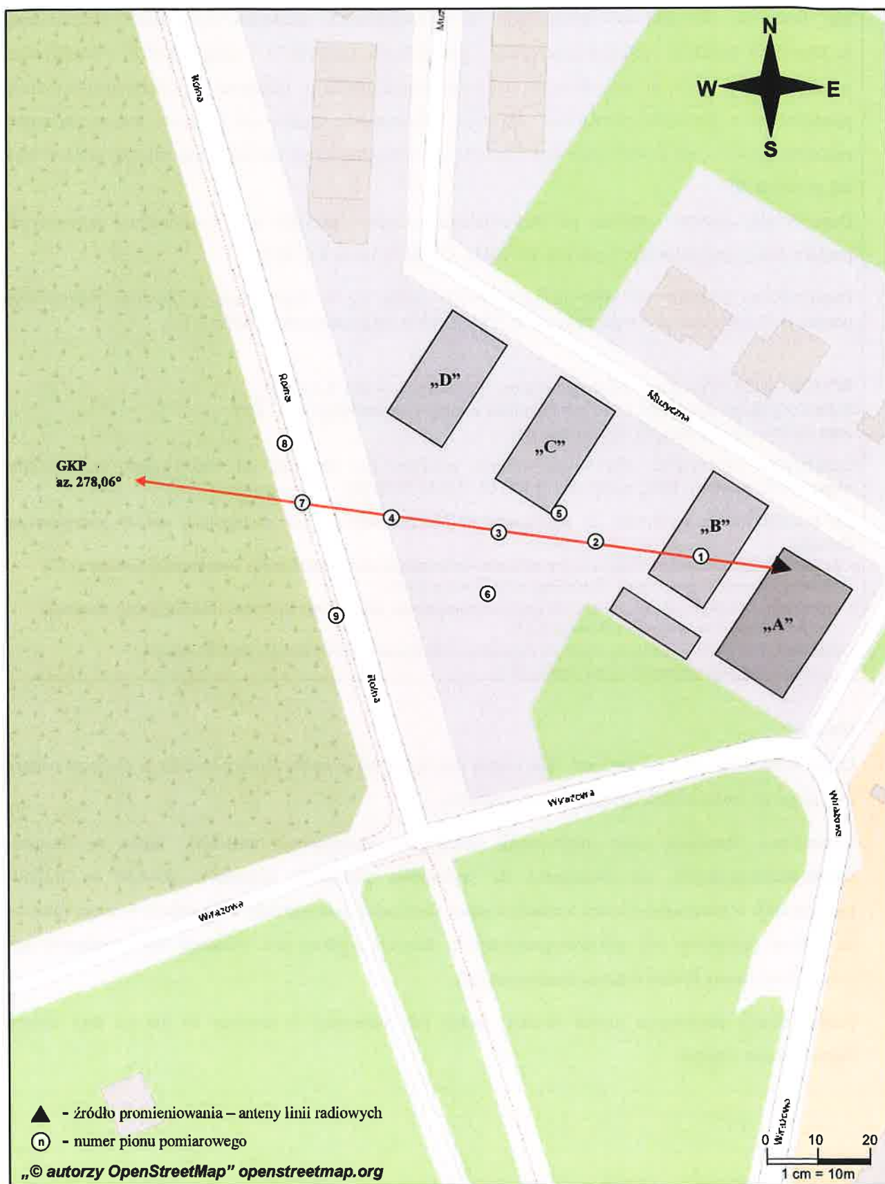
Rys. 1. Usytuowanie punktów i pionów pomiarowych w otoczeniu instalacji radiokomunikacyjnej Stacja Netia LESAB074-LESAM00025 Łazy, ul. Muzyczna 26
