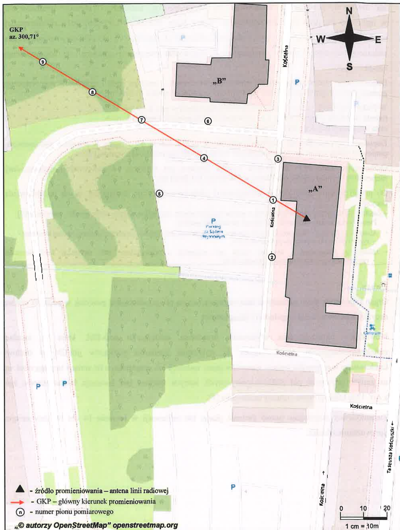
Rys. 1. Usytuowanie punktów i pionów pomiarowych w otoczeniu instalacji radiokomunikacyjnej Stacja Netia PIASB033-PIASM00033 Piaseczno, ul. gen. Tadeusza Kościuszki 14
