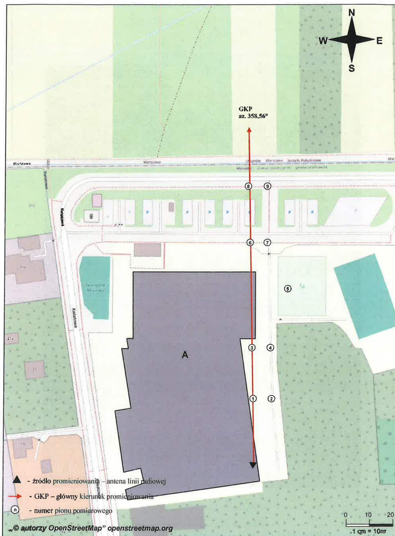
Rys. 1. Usytuowanie punktów i pionów pomiarowych w otoczeniu instalacji radiokomunikacyjnej Stacja Netia LESAB037-LESAM00020 Mysiadło, ul. Kwiatowa 28
