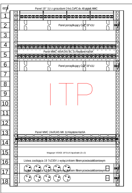
Szafa C&C wisząca niedzielona 18U 600x400mm
