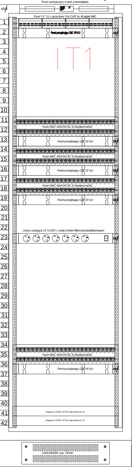
Szafa C&C 42U 600x800x2030 nośność 400kg RAL 9005
