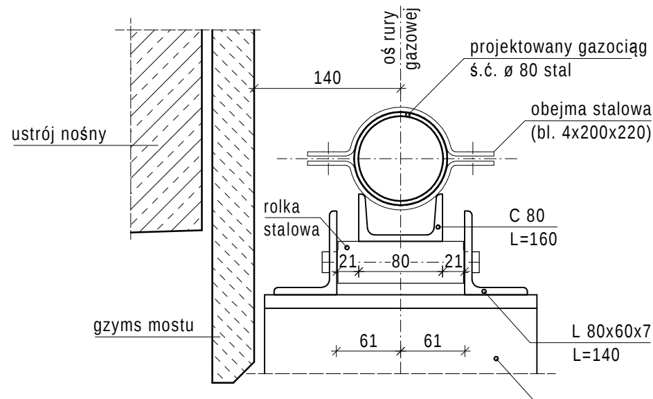
SZCZEGÓŁ "S1" SKALA 1:5
