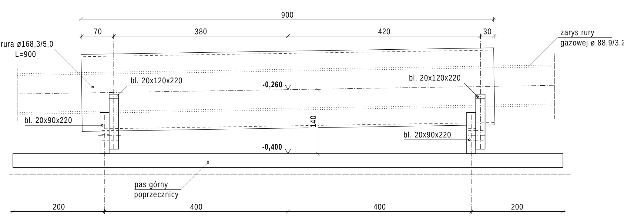
SZCZEGÓŁ "S2" SKALA 1:5
