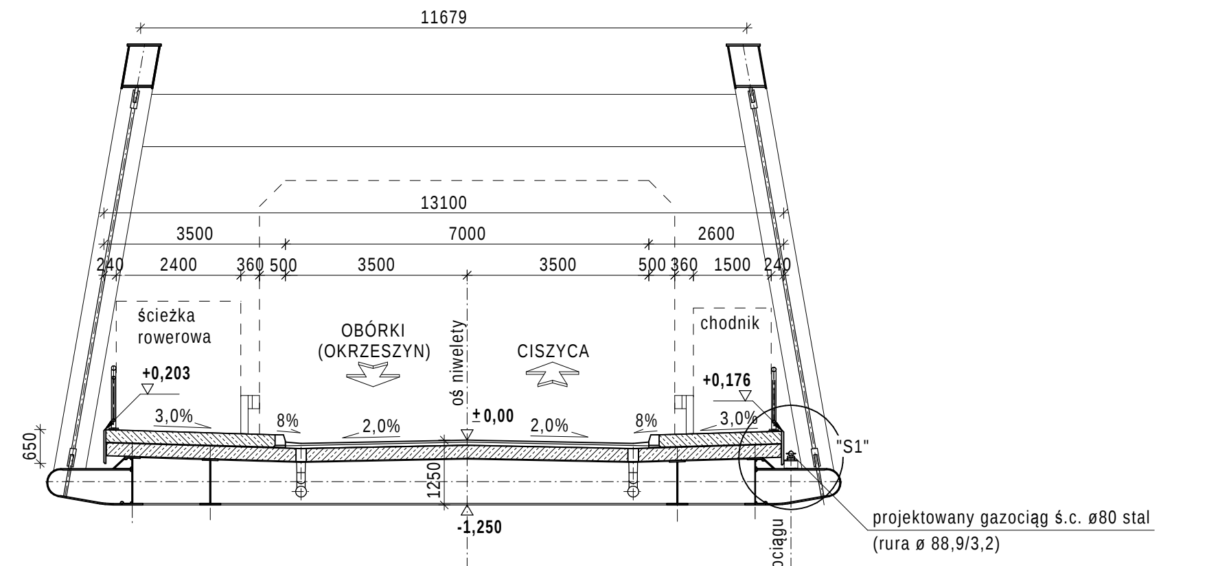
PRZĘKROJE SKALA 1:100 PRZĘKROJ PRZĘSŁOWY
