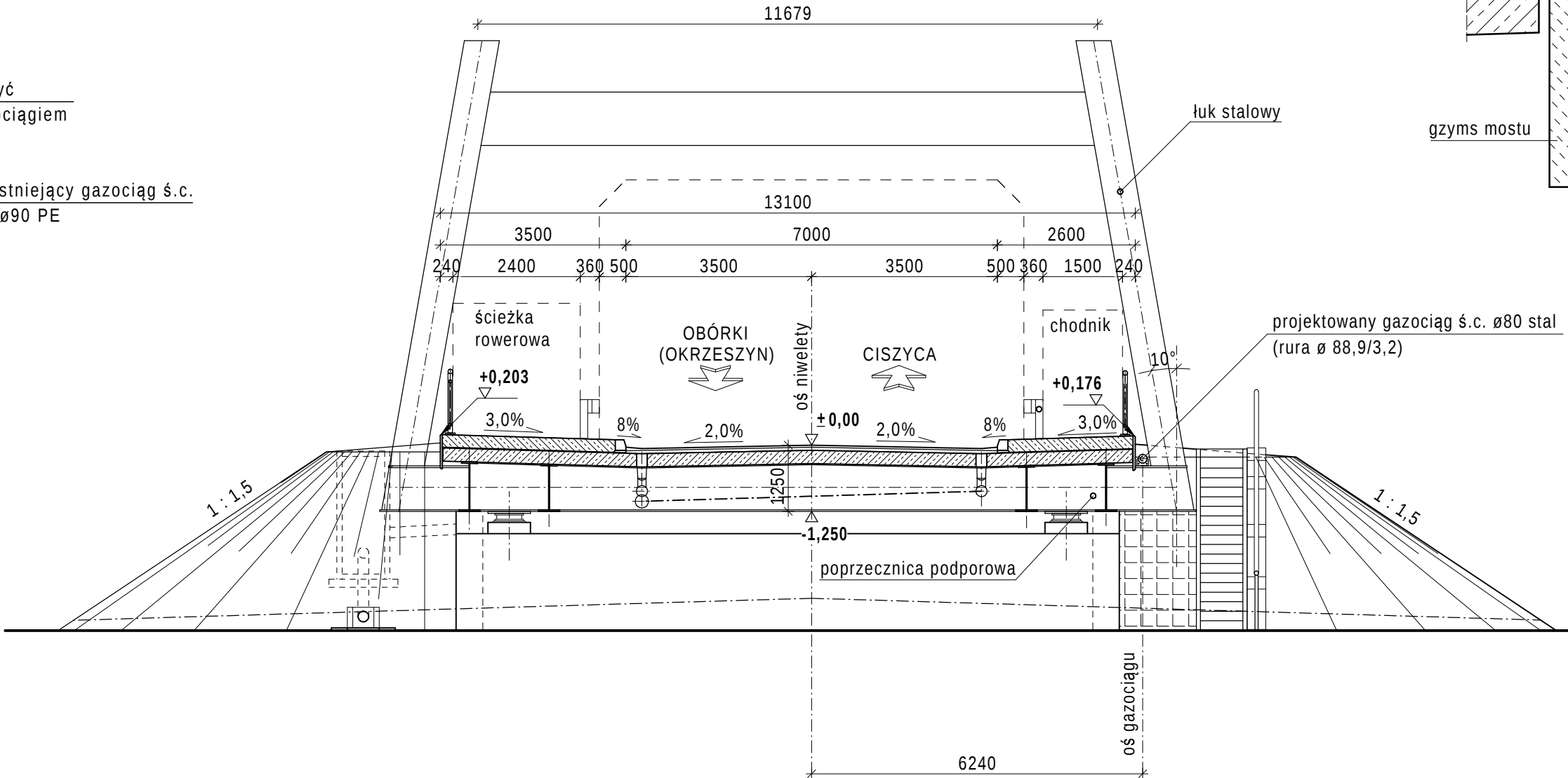
PRZĘKROJ PODPOROWY
