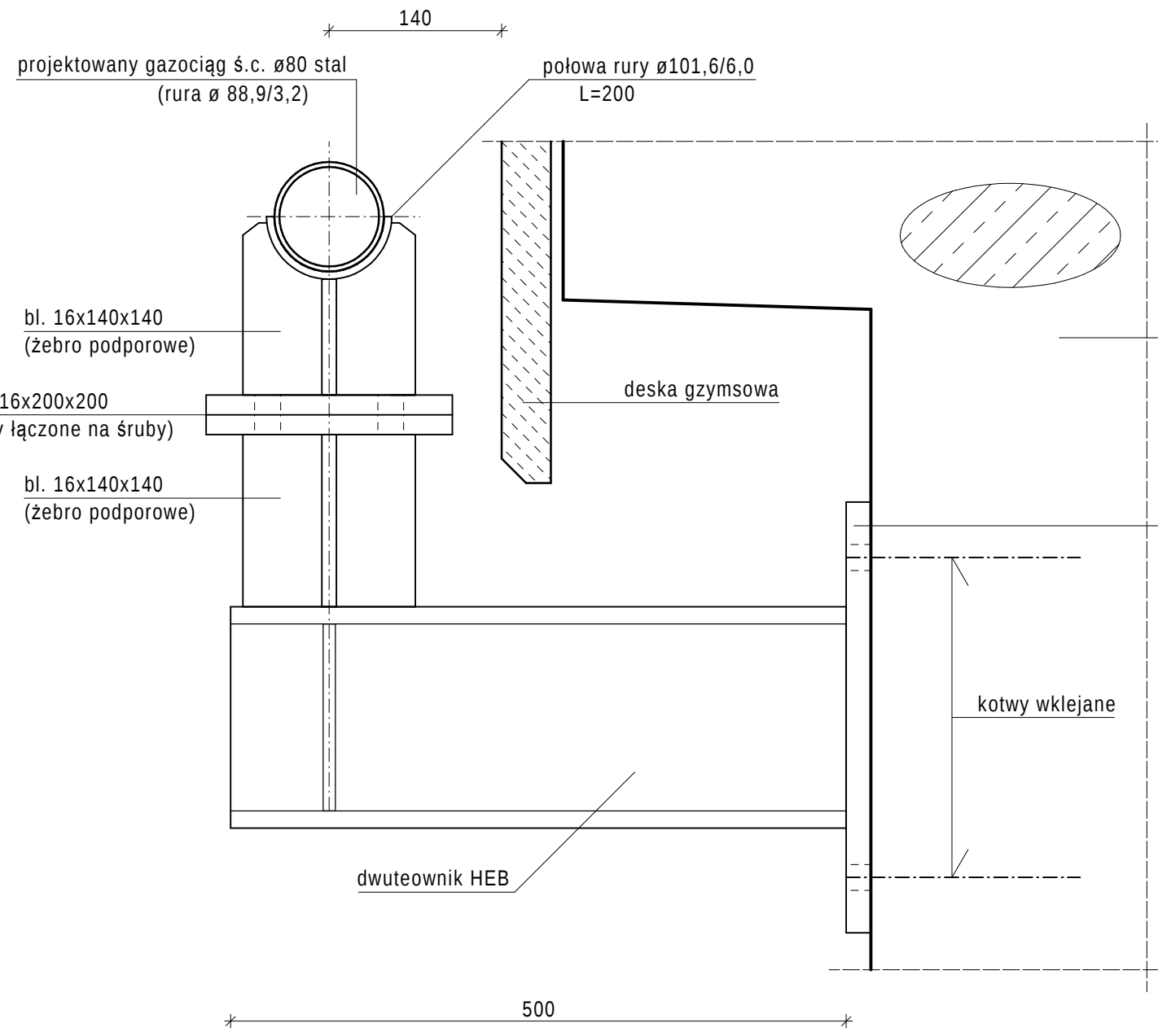
PUNKT STAŁY SKALA 1:5
