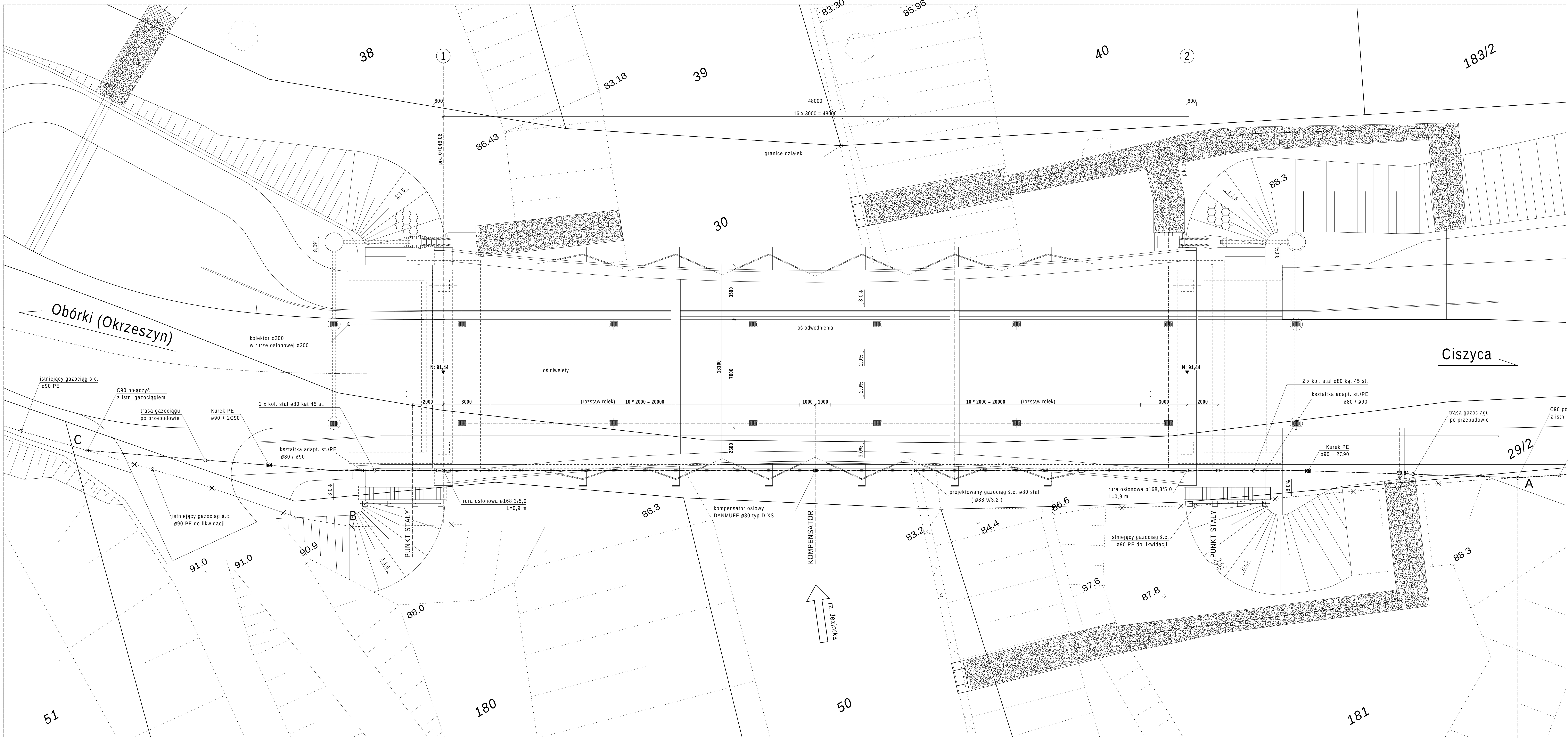
WIDOK Z GÓRY SKALA 1:100
