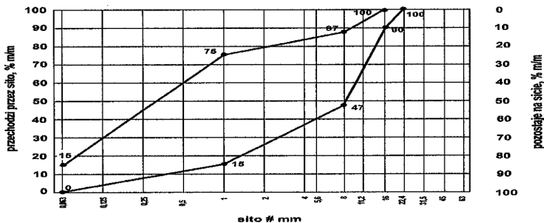
Rys. Uziarnienie mieszanki niezwiązanej 0/16 dla nawierzchni
