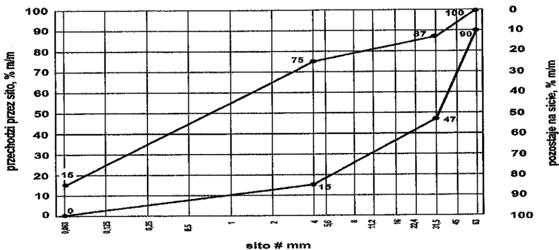
Rys. Uziarnienie mieszanki niezwiązanej 0/63 dla nawierzchni
