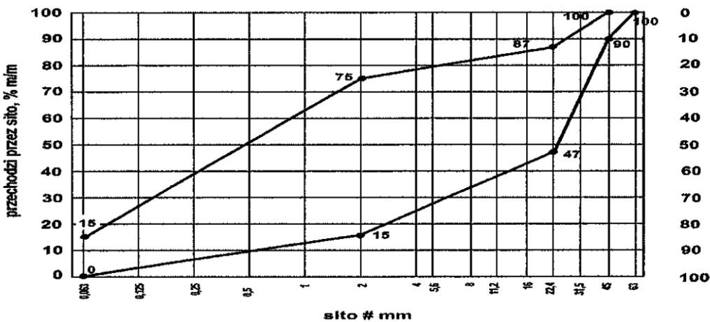
Rys. Uziarnienie mieszanki niezwiązanej 0/45 dla nawierzchni
