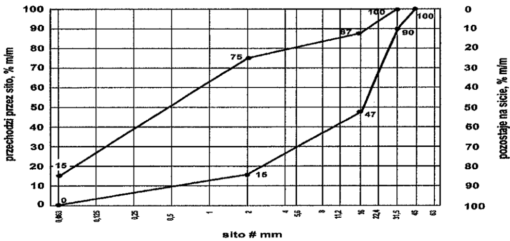
Rys. Uziarnienie mieszanki niezwiązanej 0/31,5 dla nawierzchni
