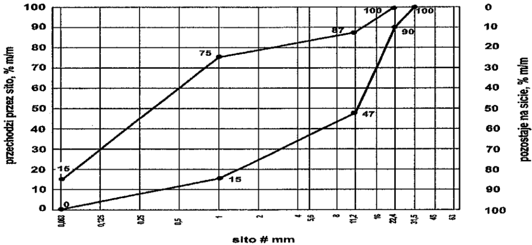
Rys. Uziarnienie mieszanki niezwiązanej 0/22,4 dla nawierzchni
