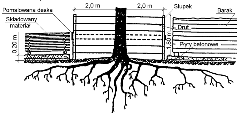
Rys. 6. Przykład ekologicznego zabezpieczenia drzewa z bryłą korzeniową na placu składowym (wg [2])
