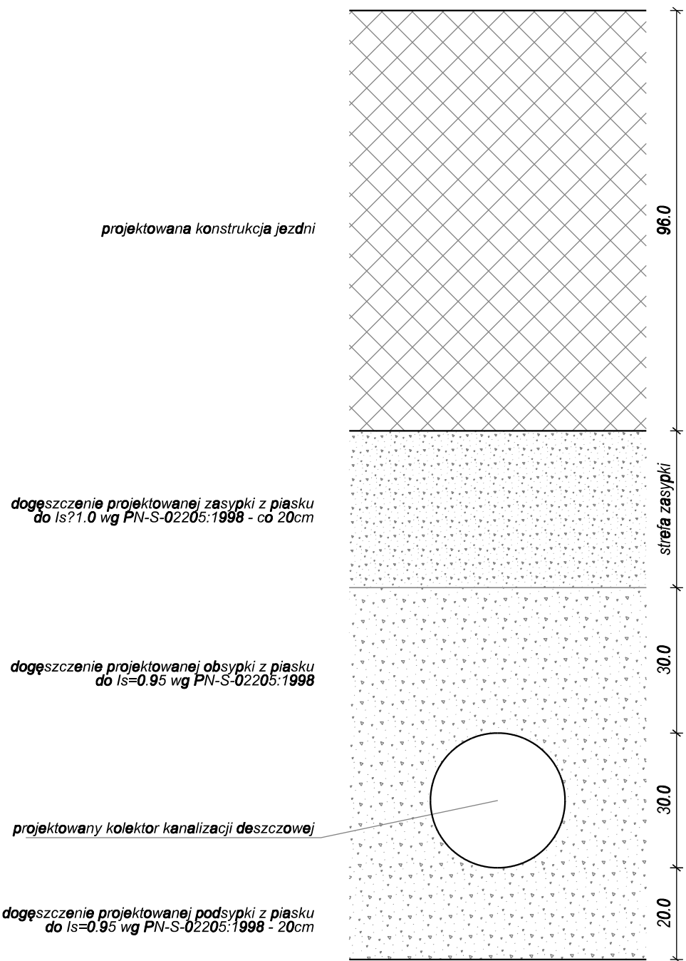
przekrój wykopu pod kanał deszczowy
