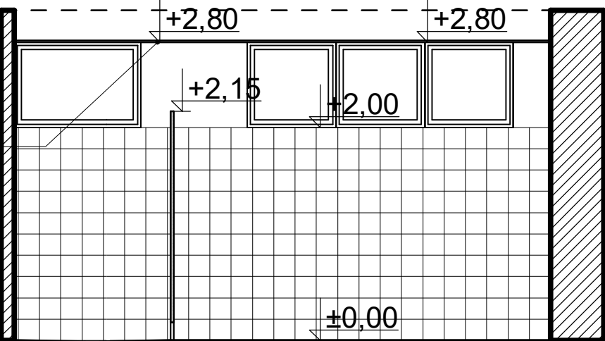
WIDOK ŚCIANY D-D
