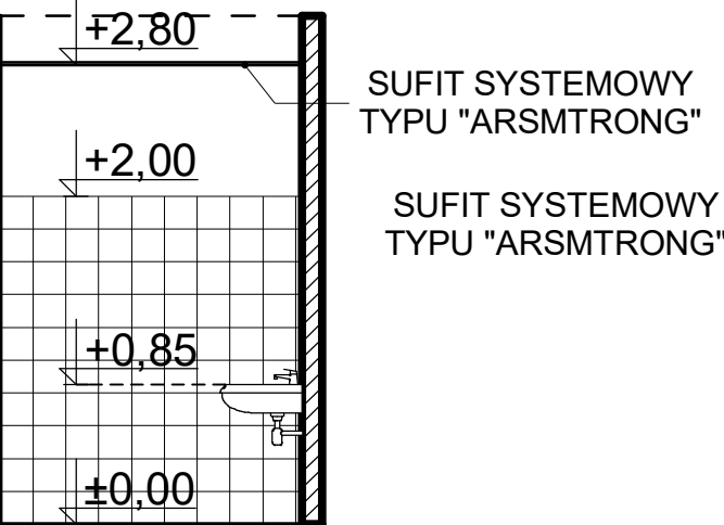
WIDOK ŚCIANY A-A
