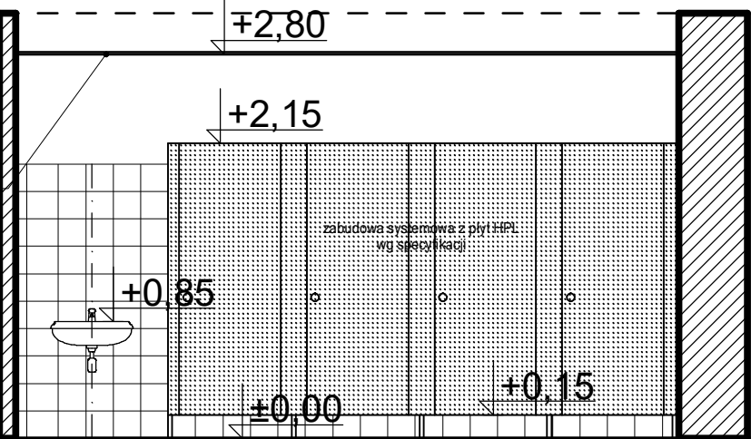
WIDOK ŚCIANY B-B
