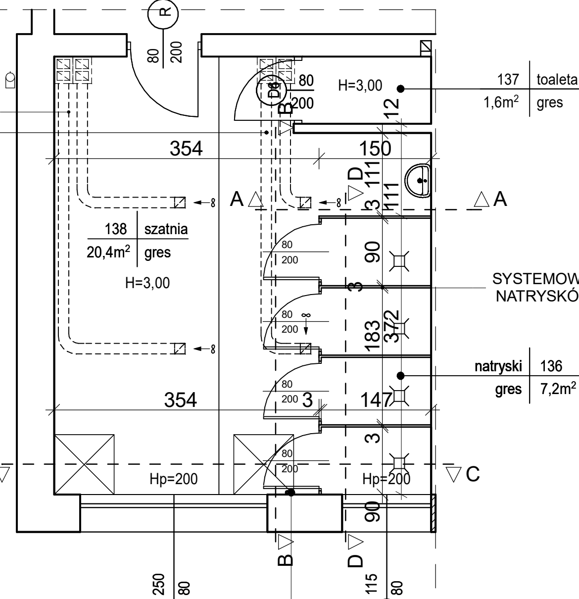
RZUT NATRYSKÓW, SZARNI I TOALETY - STAN PROJEKTOWANY
