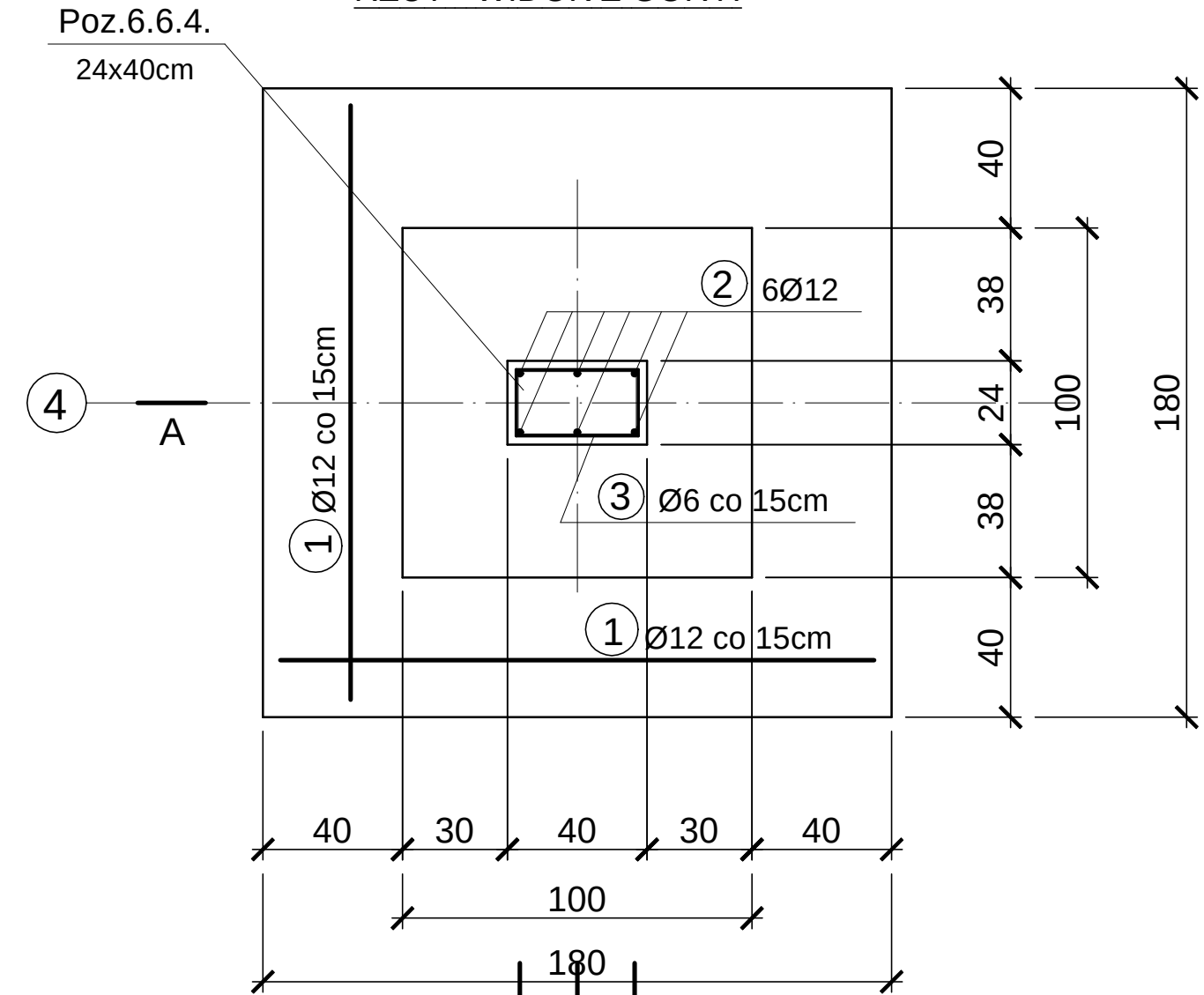
RZUT - WIDOK Z GÓRY.
