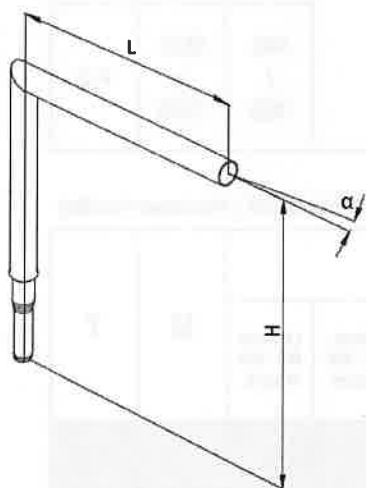
WYSIEGNIK KC BRACKET KC
